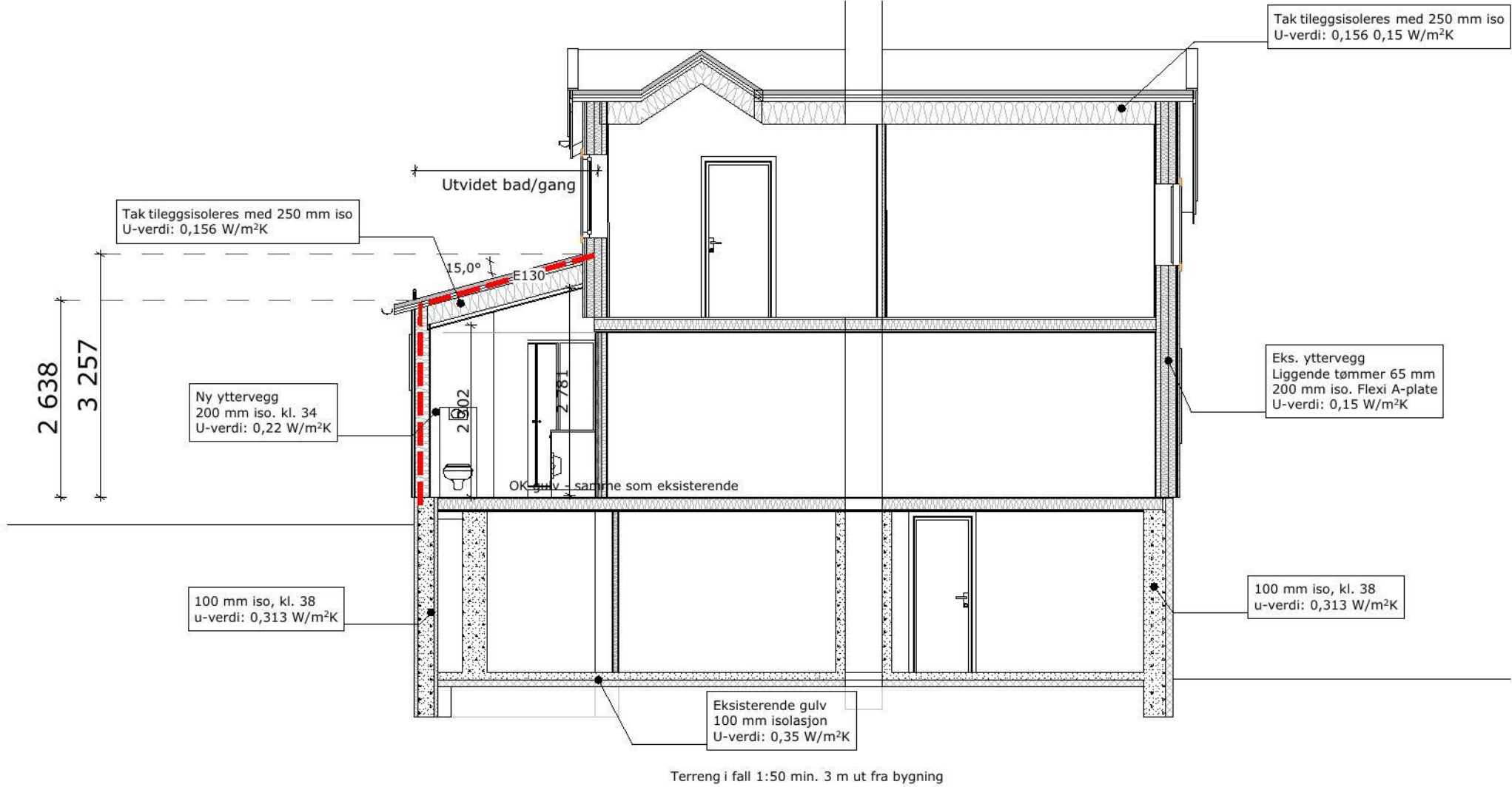
Snitt B
