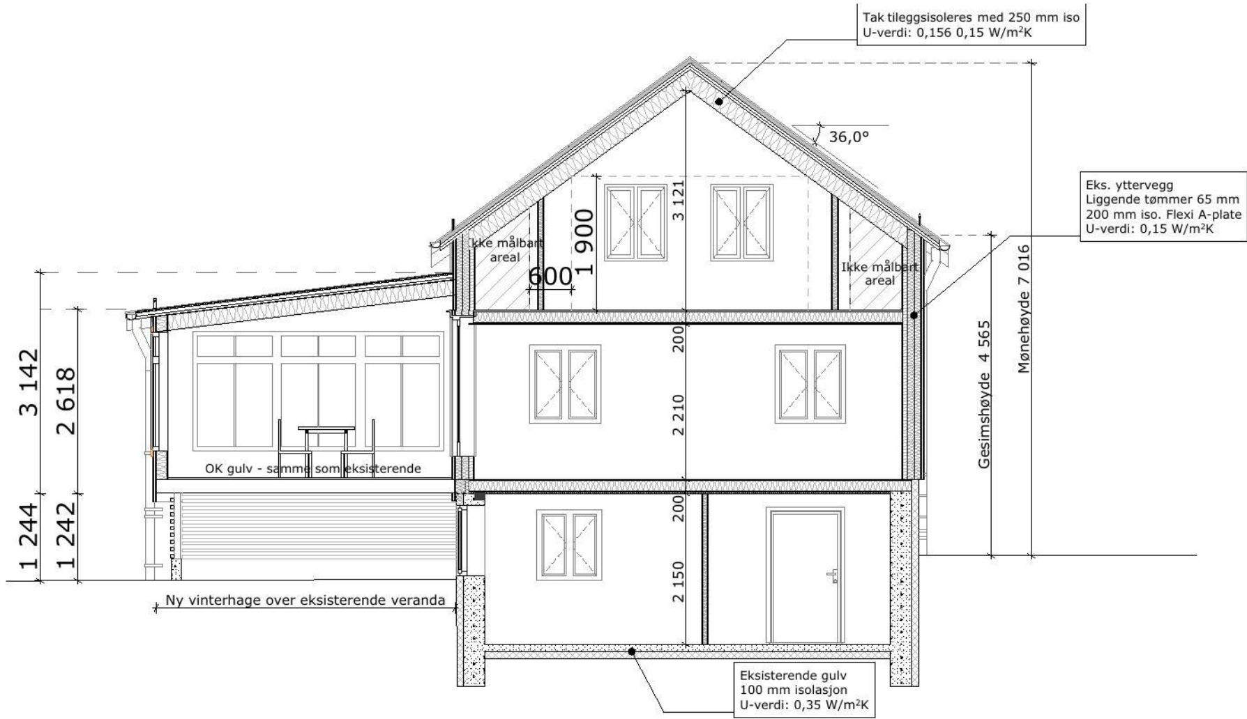
Snitt A
